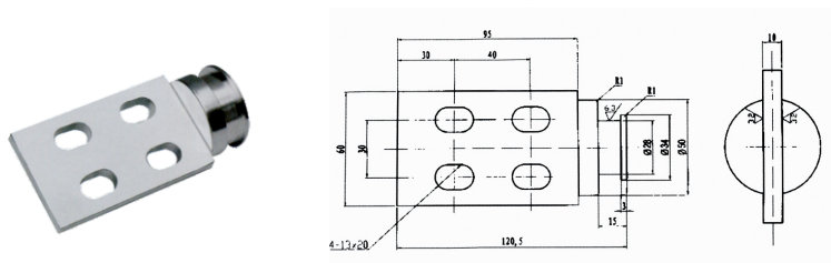
ZN85-40.5/630A 隔离触臂 材料：紫铜 产品编号：ZH038
