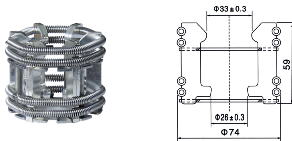
GC5-630A/1000A 捆绑式触头 触片数量: 12 片 产品编号: ZH010
