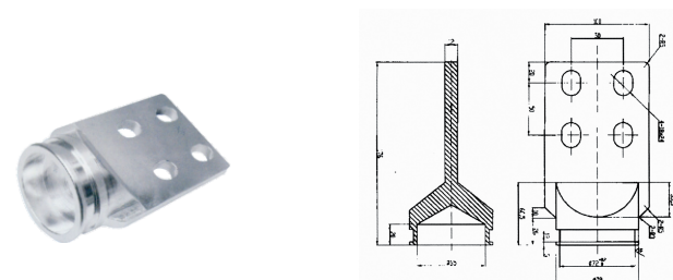
ZN85-40.5/2000A 隔离触臂 材料：紫铜 产品编号：ZH041
