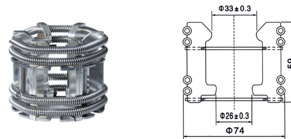
GC5-630A/1000A 捆绑式触头 触片数量: 12 片 产品编号: ZH012
