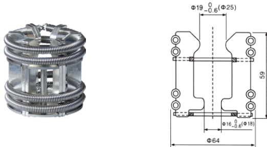
GC5-630A 捆绑式触头 触片数量: 12 片 产品编号: ZH009
