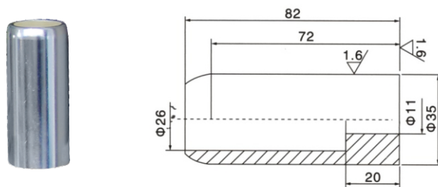
630A 静触头 材料：紫铜 / 铜铝焊接 产品编号：ZH001
