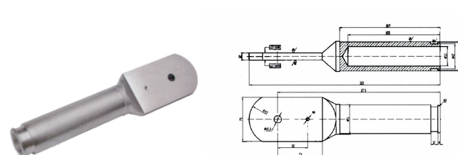
ZN94B/1250A 上触臂 材料：紫铜 产品编号：ZH044
