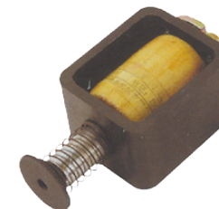
CT19分合闸磁合线圈总成
