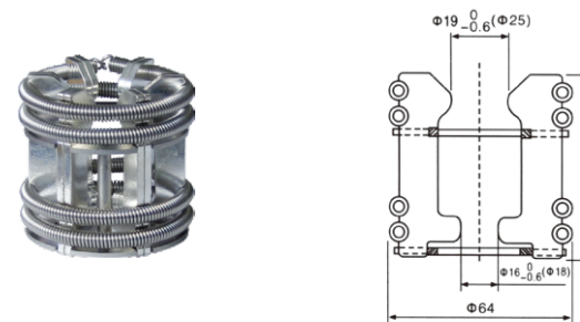
GC5-630A 捆绑式触头 触片数量: 12 片 产品编号: ZH011
