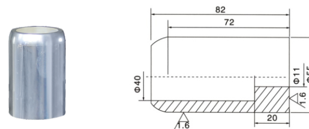
1600A 静触头 材料：紫铜 产品编号：ZH003
