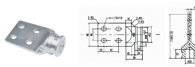
ZN85-40.5/1600A 隔离触臂 材料: 紫铜 代号: TY2010-203 产品编号: ZH040
