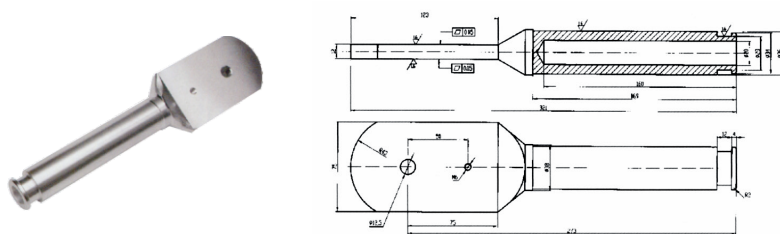
ZN94B/630A 上触臂 材料：紫铜 产品编号：ZH042
